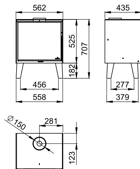
OPCIONAL P-ARUS: Patas para colocar sobre base. OPTIONAL P-ARUS: Legs to place on base. OPCIONAL P-ARUS: Pernas para colocar na base.
